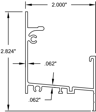
2 FRAME SILL 6063-T6 ALUMINUM
